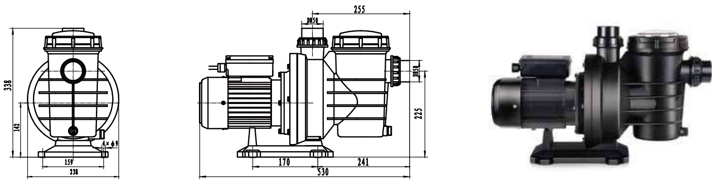
安装尺寸图
