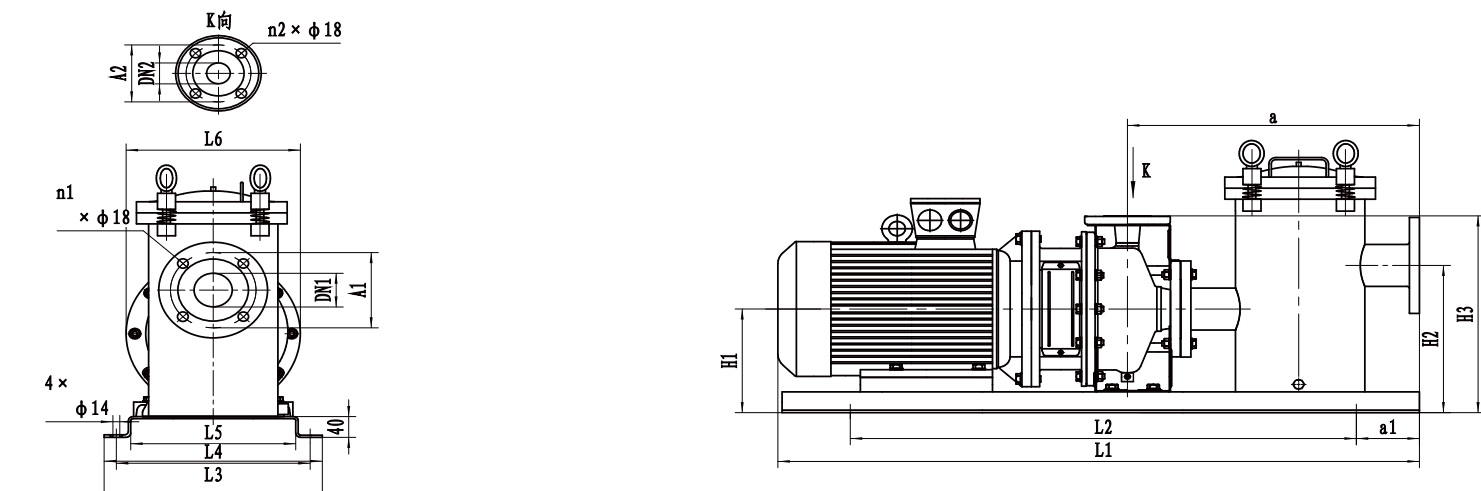
安装尺寸图
