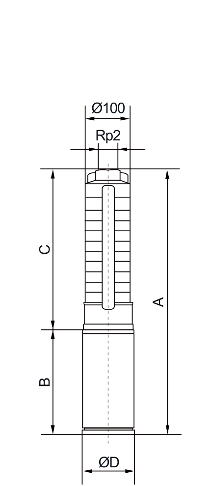
安装尺寸
