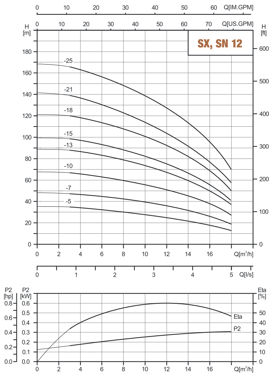
性能曲线 2850rpm
