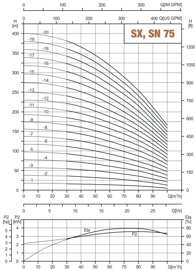
性能曲线 2900rpm
