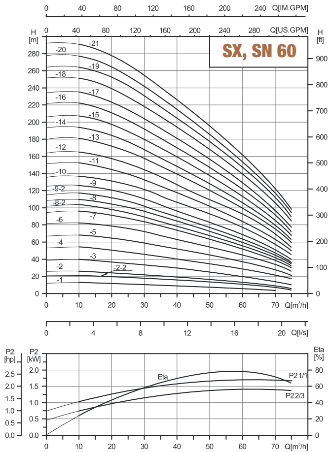
性能曲线 2850rpm
