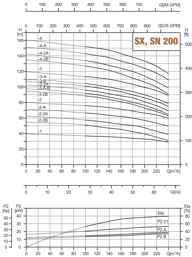
性能曲线 2900rpm
