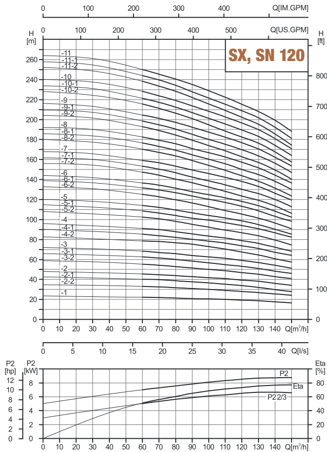
性能表
