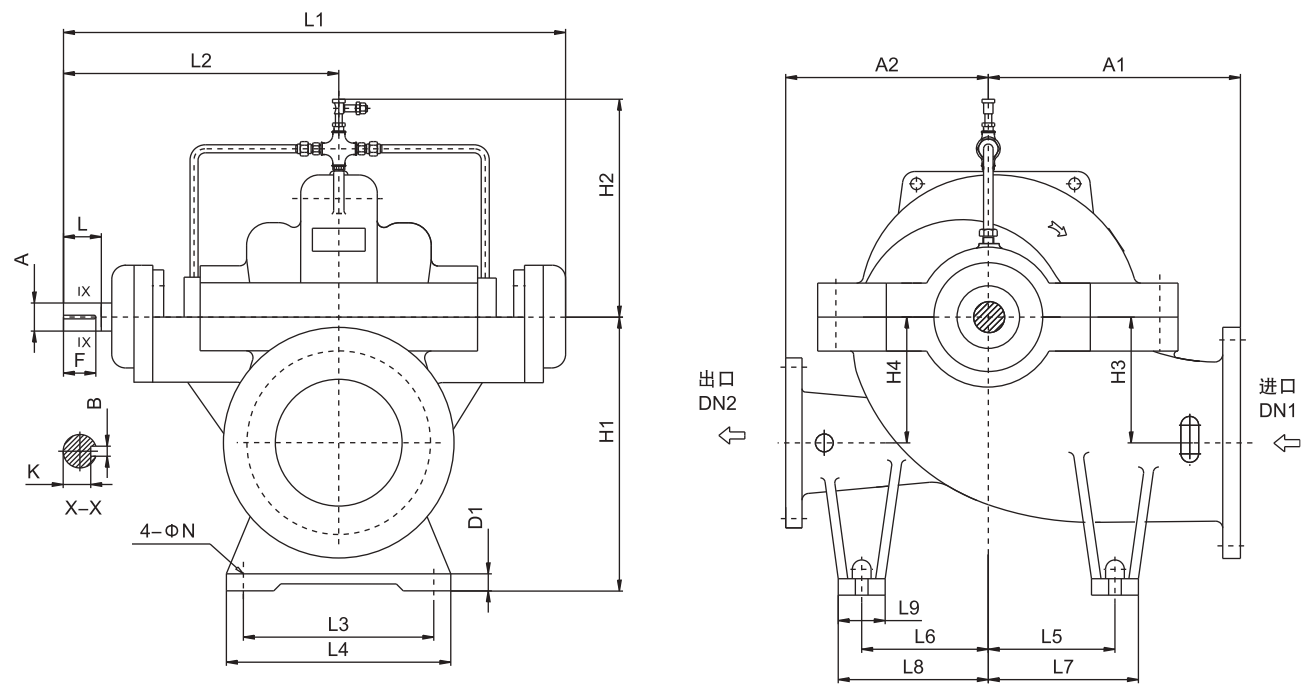
单泵主要外形尺寸
