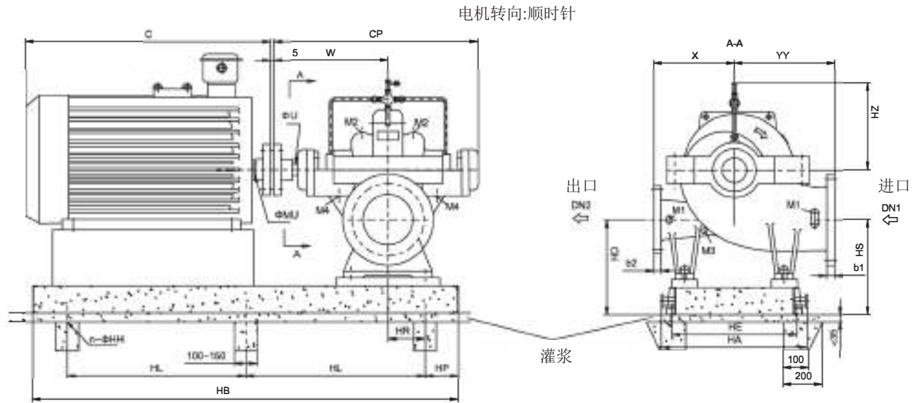
卧式安装泵组主要外形尺寸
